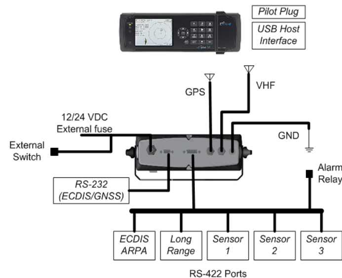
System Overzicht
